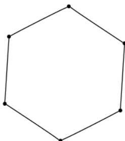
Slika 6 - ljuska grafa sa 6 čvorova; istodobno i 2-regularan graf
