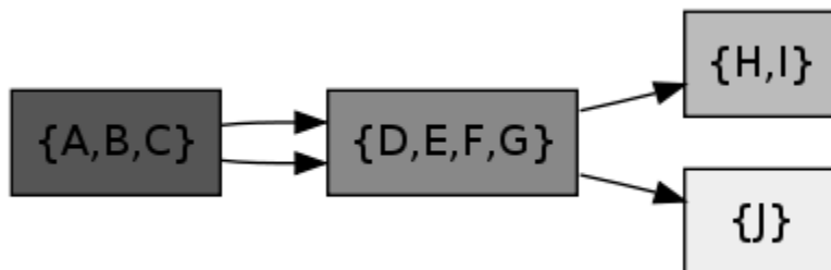
Slika 11 - kada bismo komponente grafa sa slike 10 prikazali kao čvorove, dobili bismo ovaj usmjereni aciklički graf
