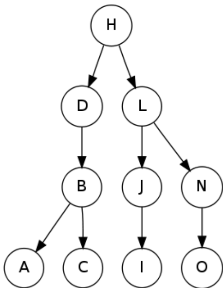
Slika 15 - primjer binarnog stabla
