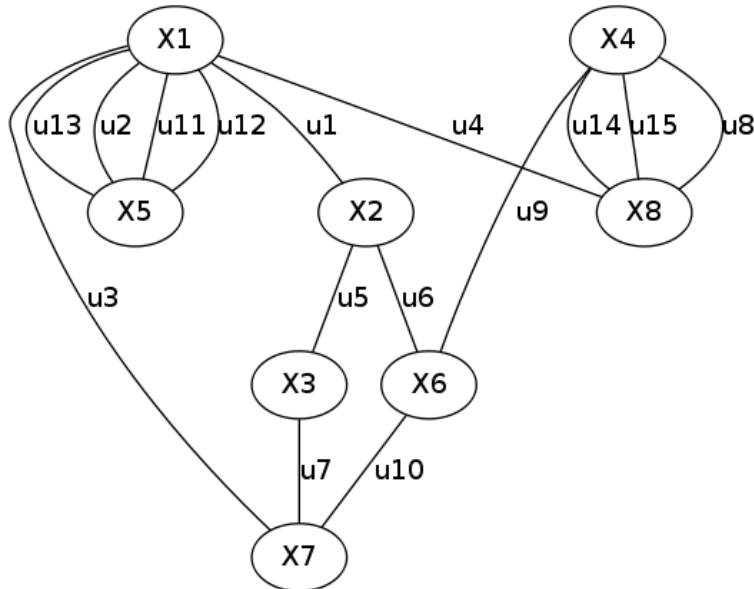
Slika 3 - Primjer multigrafa
